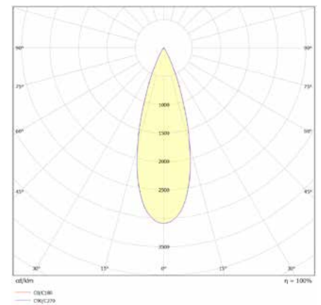
Curva polare Polar curve Ottica 36° Optics
