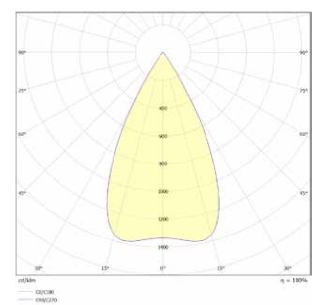
Curva polare Polar curve Ottica 60° Optics
