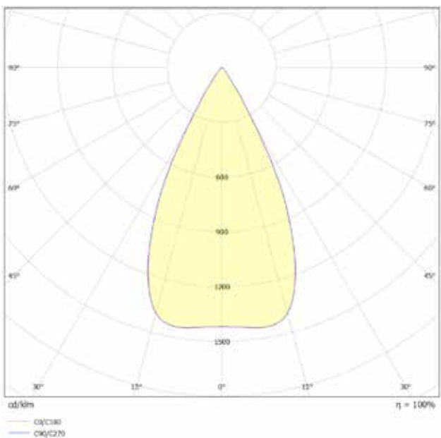
Curva polare Polar curve
