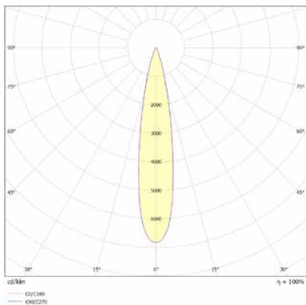
Curva polare
